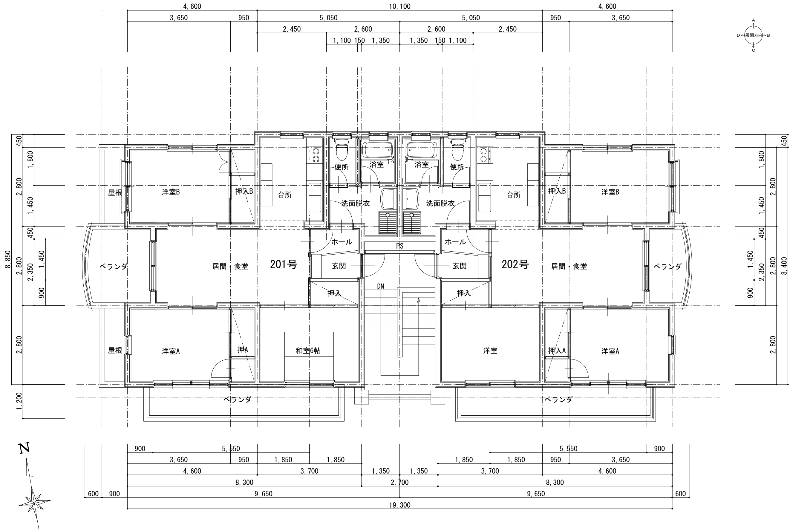
2階平面詳細図
